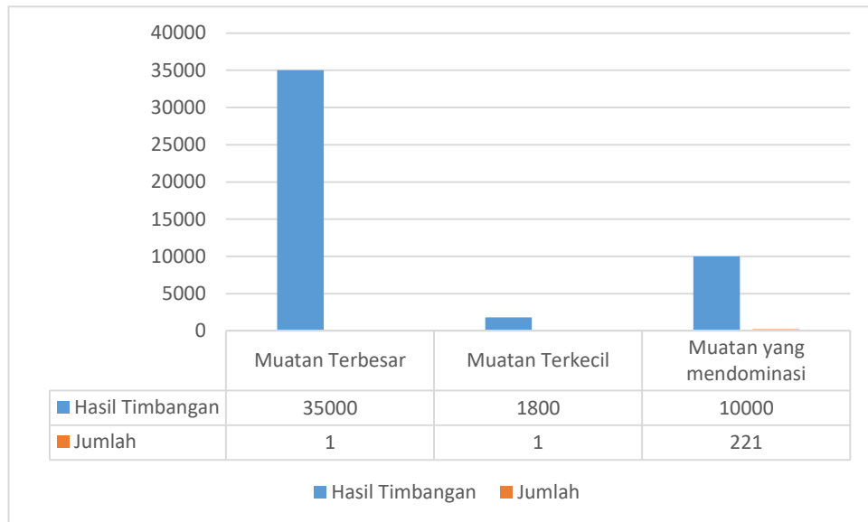
Gambar IV. 23 Data penimbangan berdasarkan muatan bulan Maret di UPPKB Merapi
