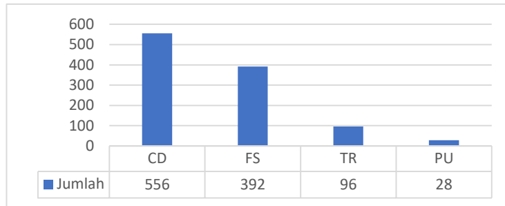
Gambar IV. 16 Jenis kendaraan terbanyak
