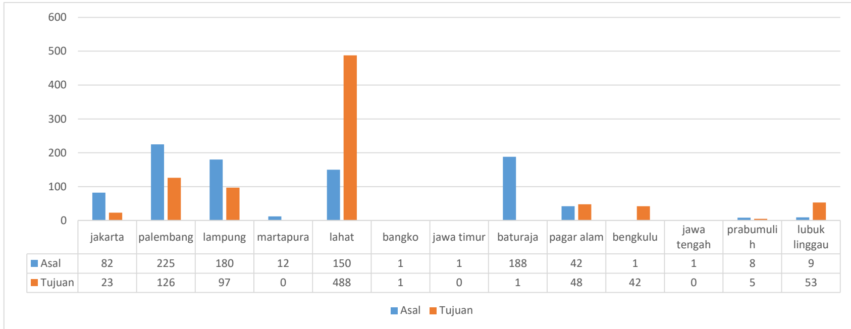
Gambar IV. 12 Asal-tujuan kendaraan angkutan barang di UPPKB Merapi
