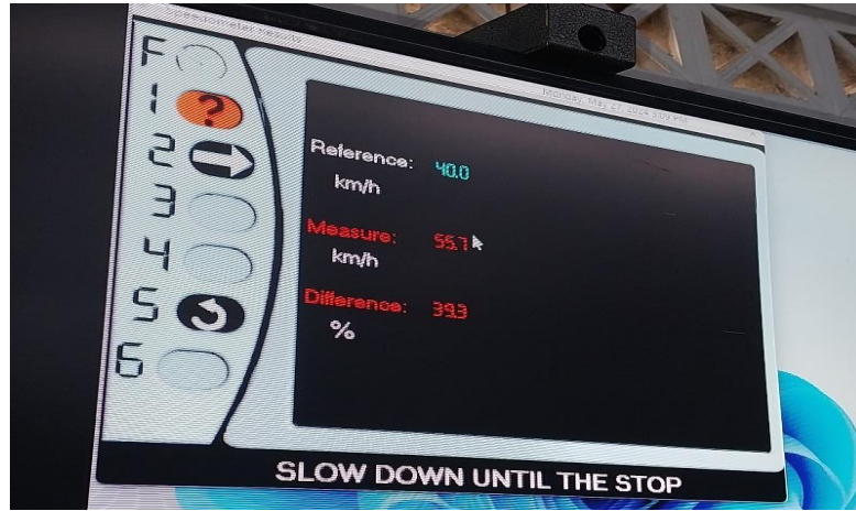
13. Display Kecepatan Pada Alat Uji Speedometer Tester (50km/jam)
